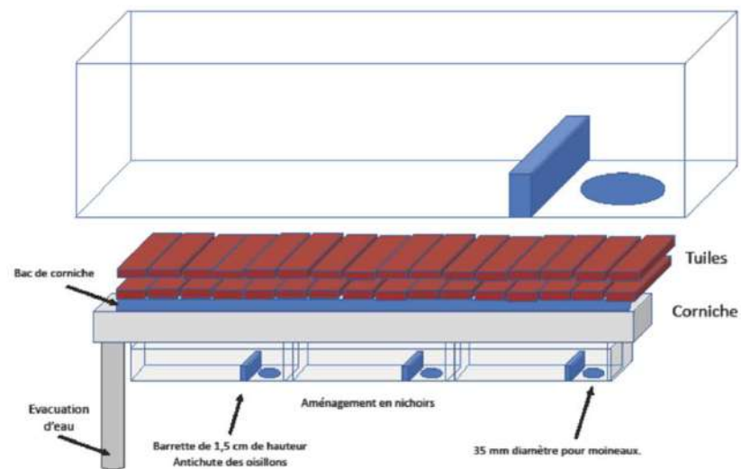
Aménagement d'une corniche (horizontale).
